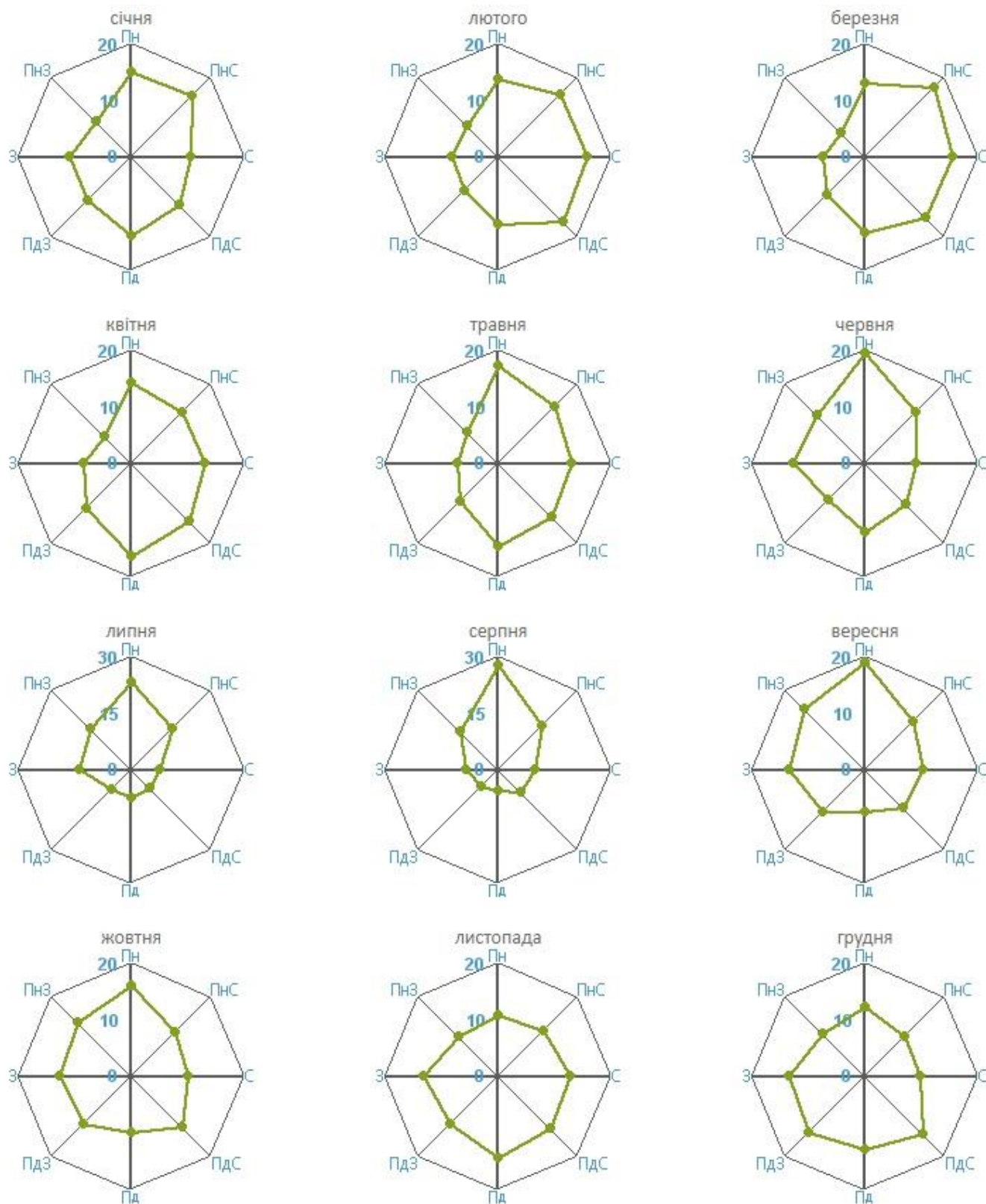
Рис.13.16.6. Повторюваність (%) напрямку вітру та штилю
